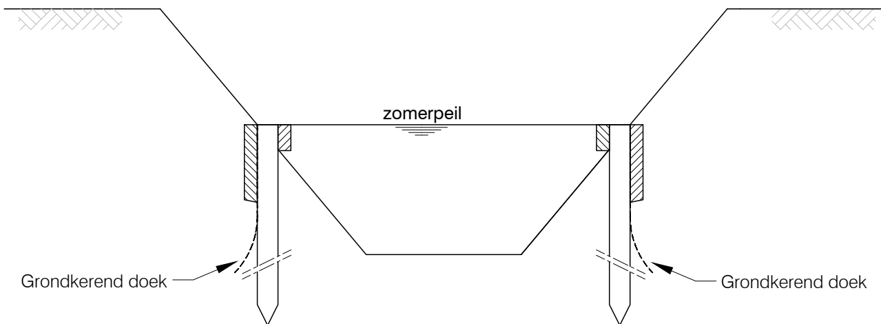
Dwarsdoorsnede
