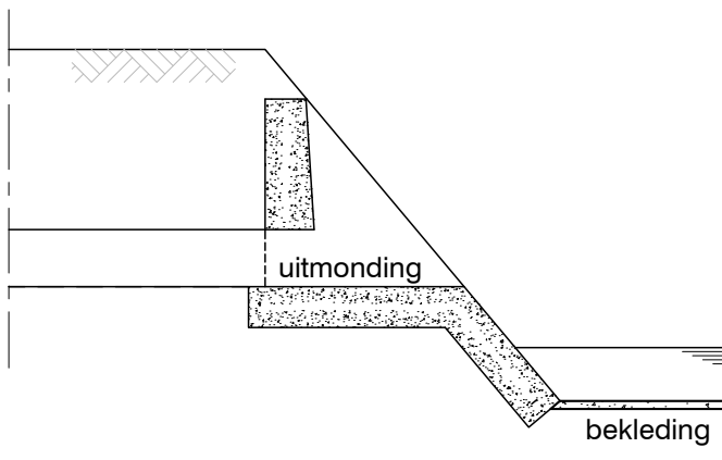
Dwarsdoorsnede A-A
