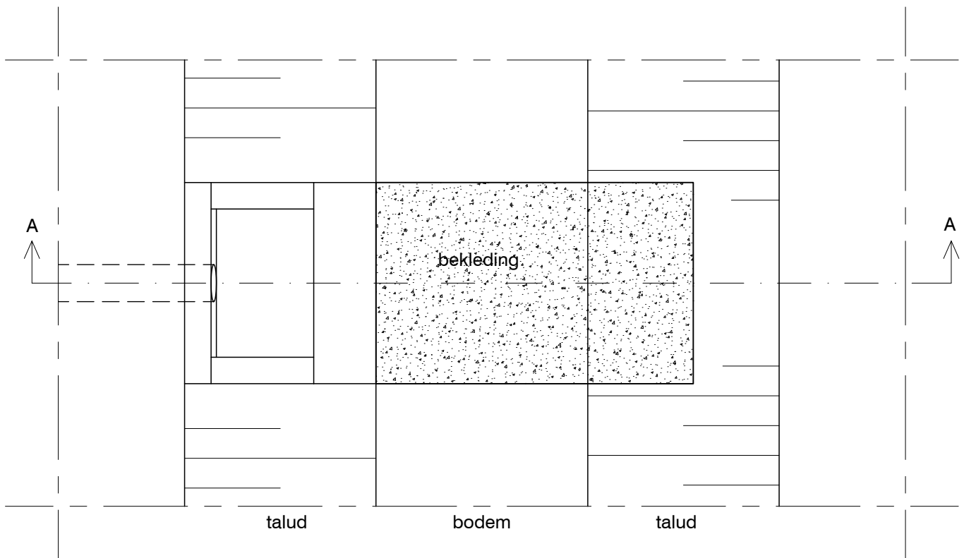
Bovenaanzicht
