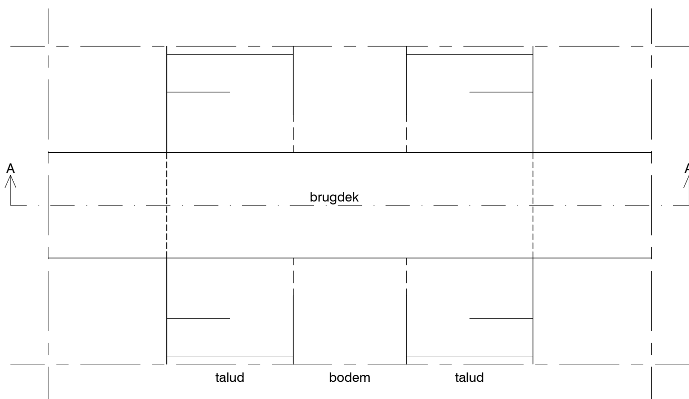
Bovenaanzicht
