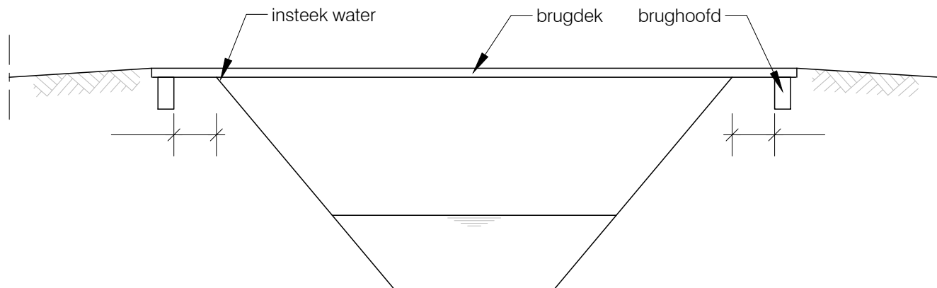
Dwarsdoorsnede A-A
